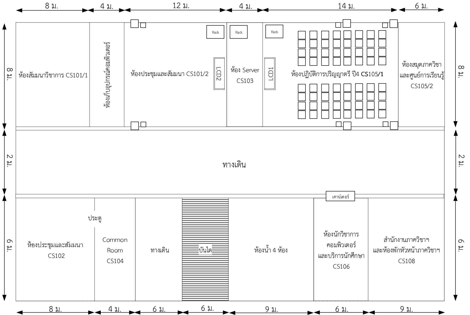
แผนผังชั้น 1 อาคารภาควิชาวิทยาการคอมพิวเตอร์
