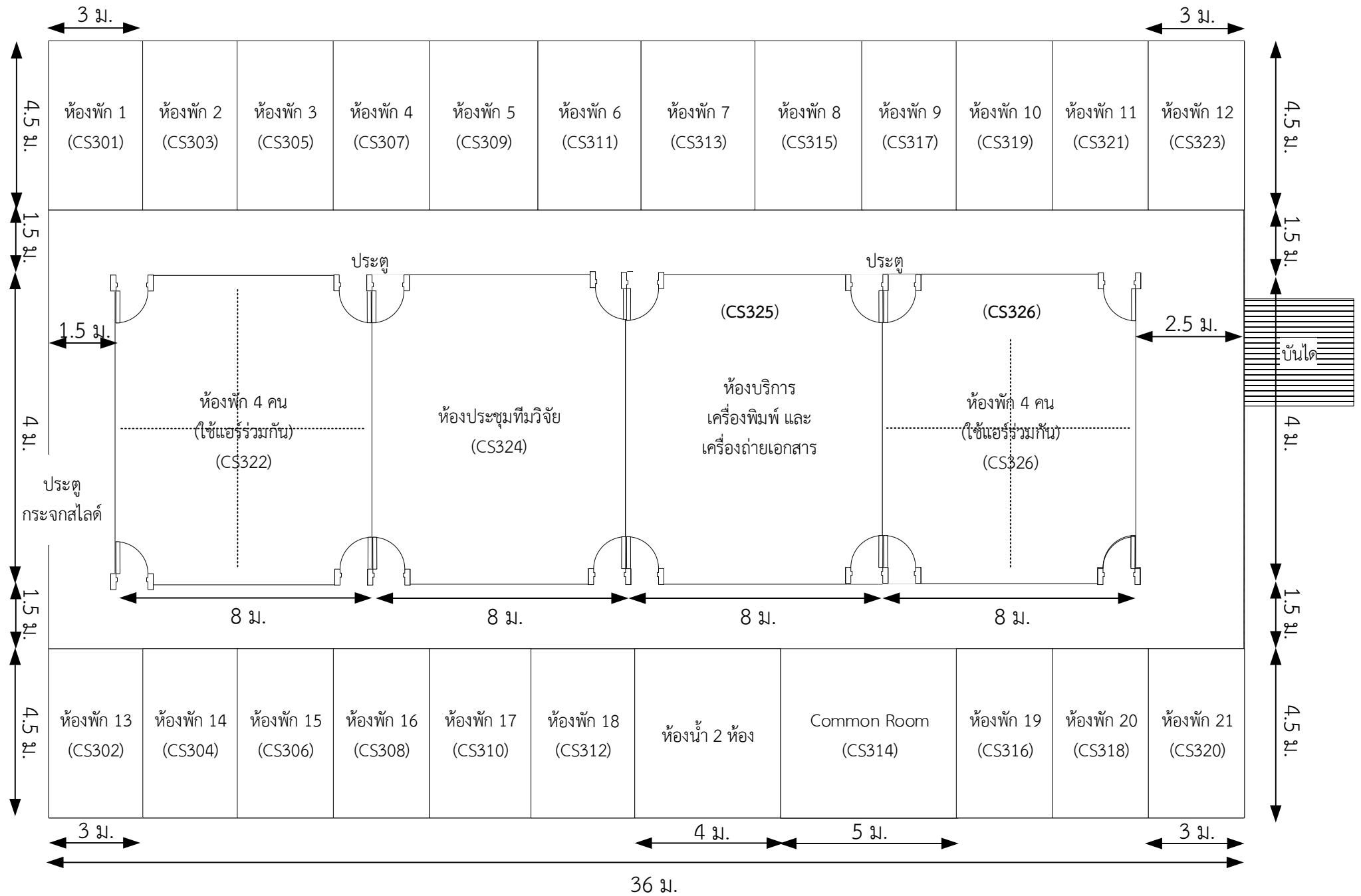
แผนผังชั้น 3 อาคารภาควิชาวิทยาการคอมพิวเตอร์
