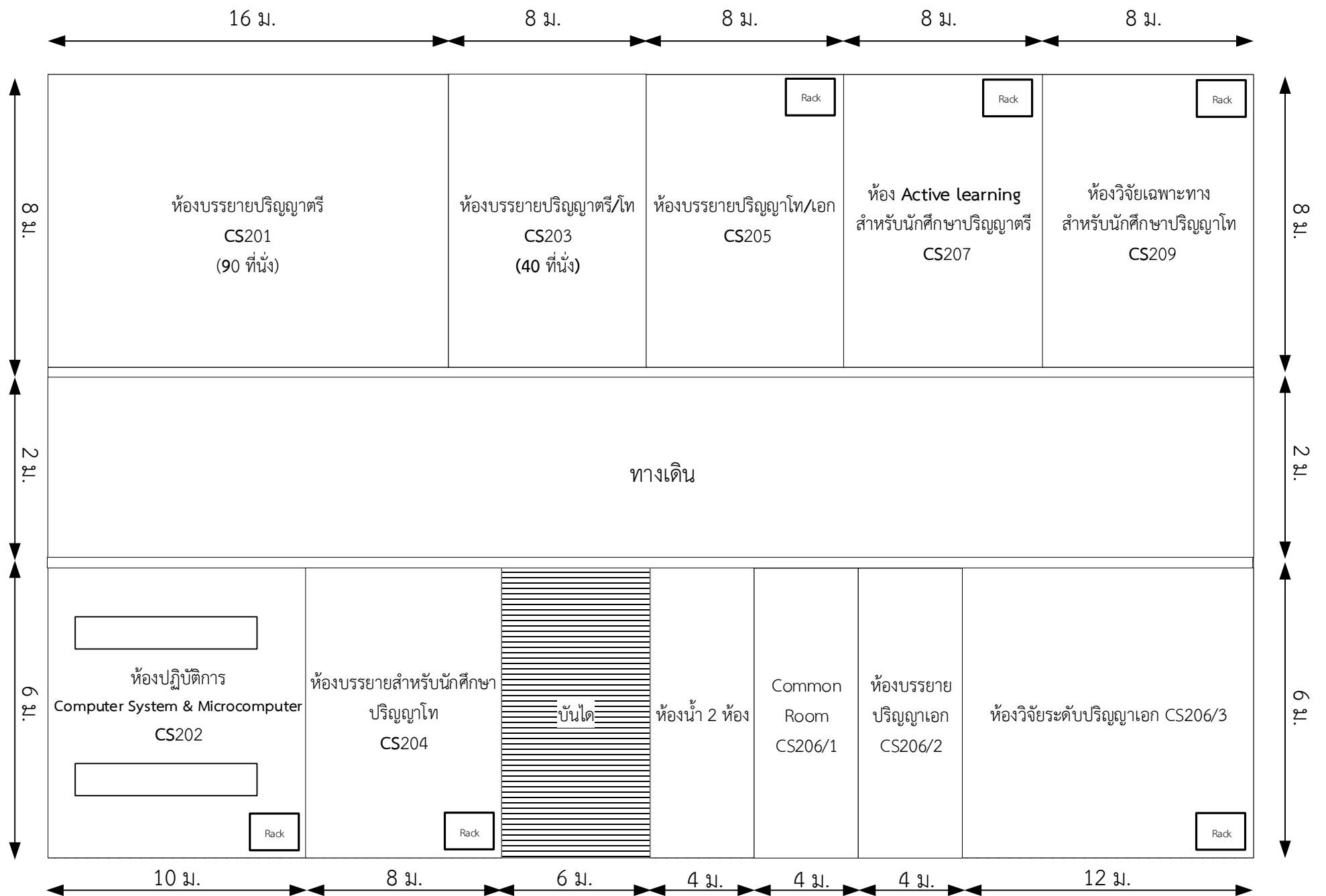
แผนผังชั้น 2 อาคารภาควิชาวิทยาการคอมพิวเตอร์
